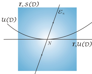
Figure 1: T_N \mathcal{S}(D) = \mathcal{E}_N^s \oplus T_N \mathcal{U}(D)
